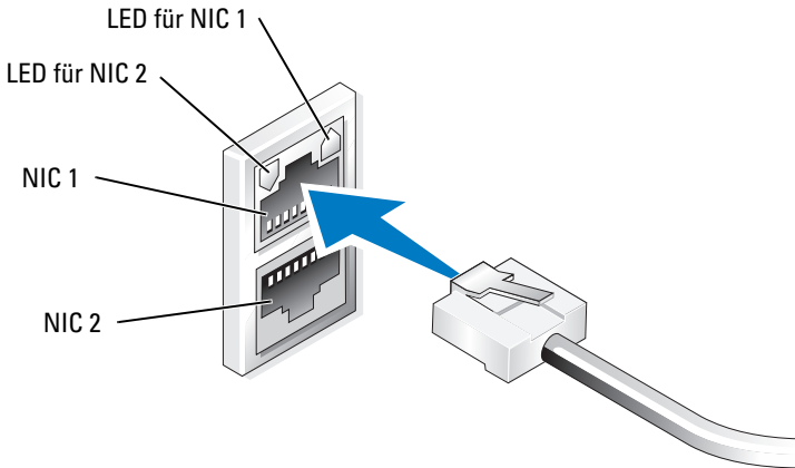
Abbildung 1-1. NIC-Anschluss
